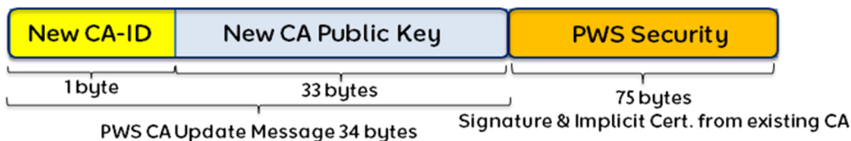
Figure 7.6.1.2 : PWS CA update message format
