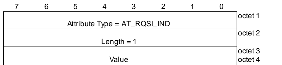
Figure 8.1.1.1-1: AT_RQSI_IND attribute
