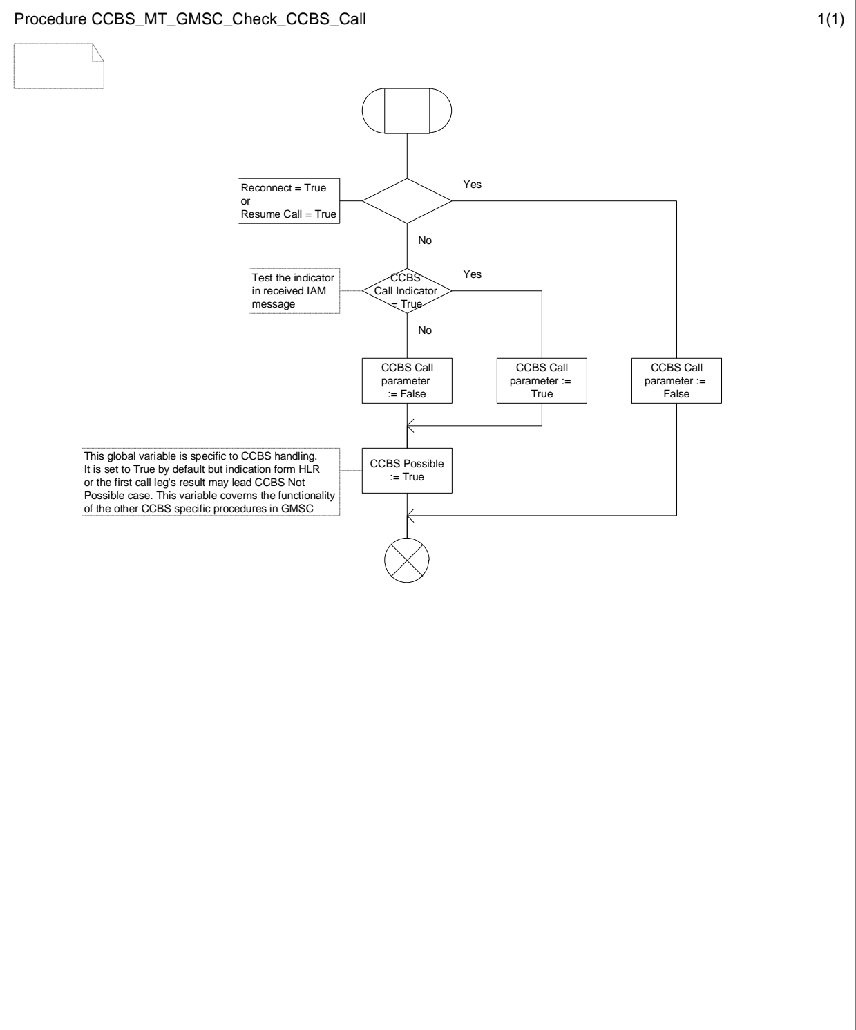
Figure 11.2.1.1: Procedure CCBS_MT_GMSC_Check_CCBS_Call
