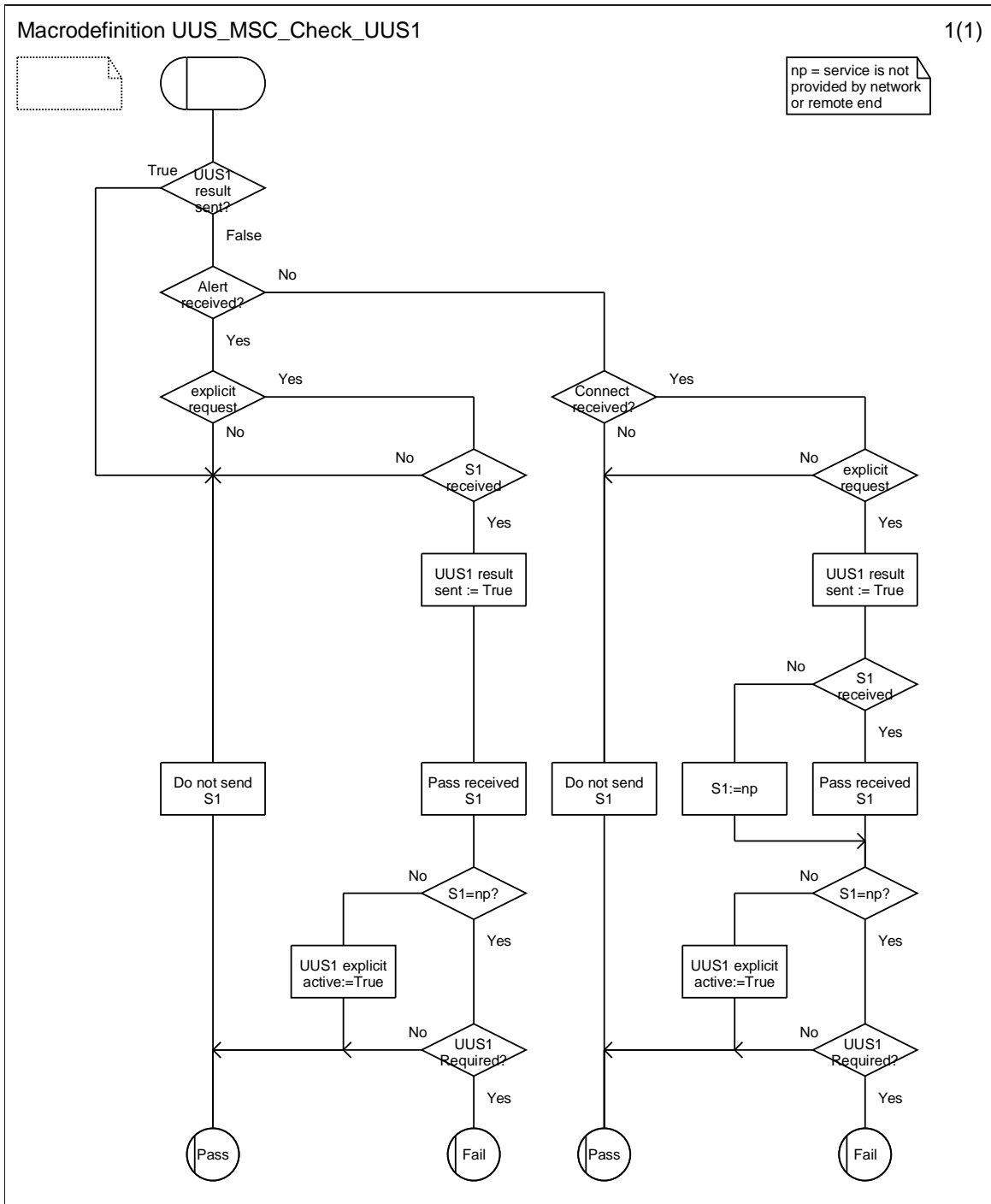
Figure 9.3.7: Macrodefinition UUS_MSC_Check_UUS1
