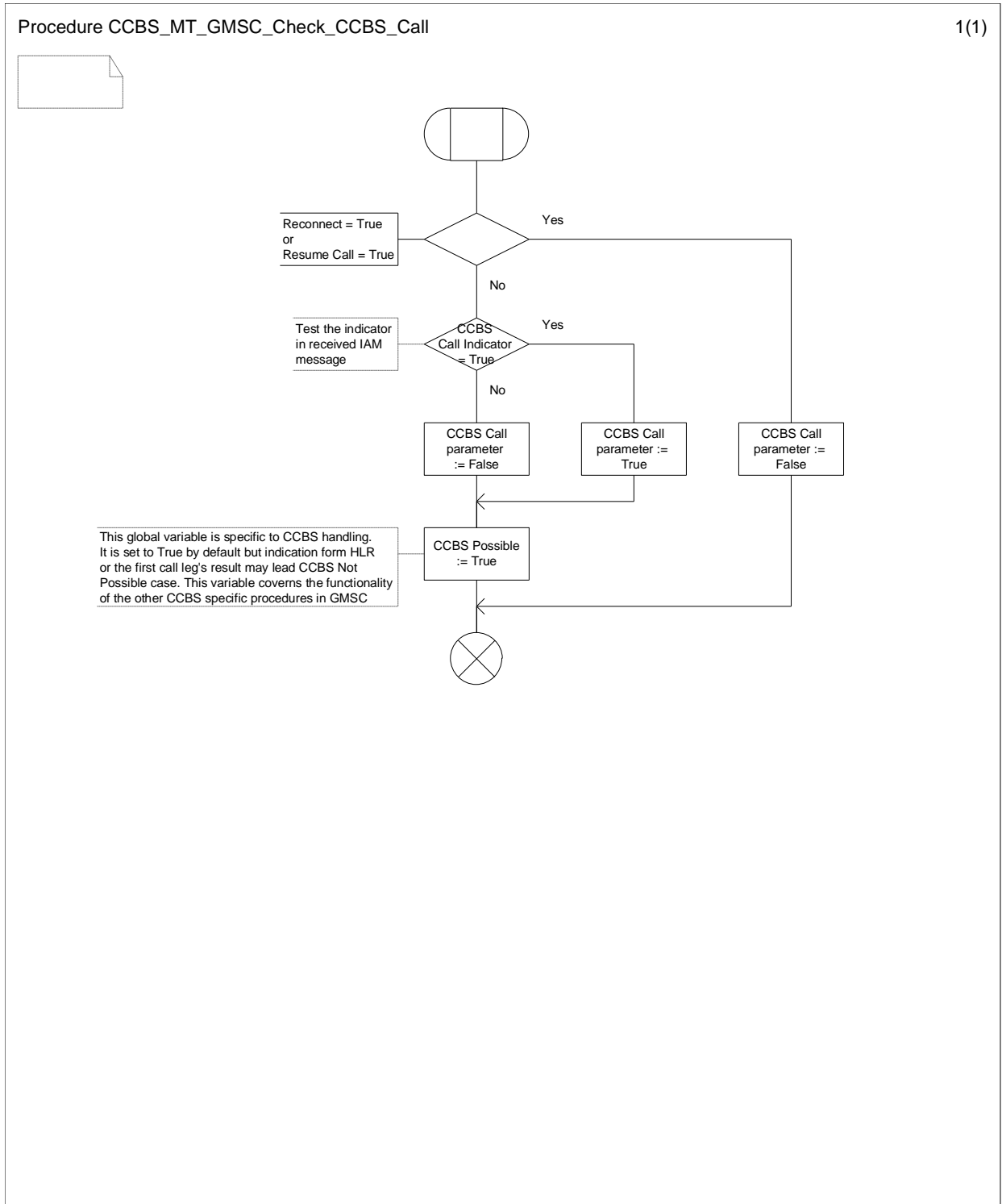
Figure 11.2.1.1: Procedure CCBS_MT_GMSC_Check_CCBS_Call
